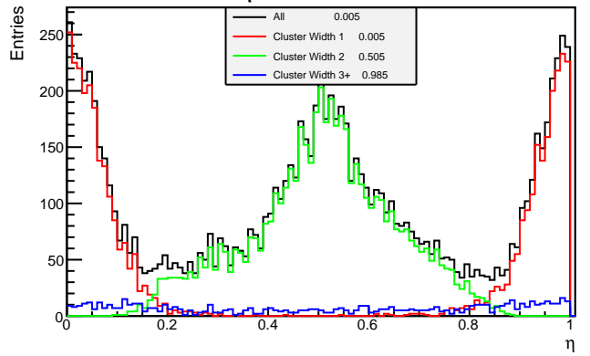
\eta -Distribution
