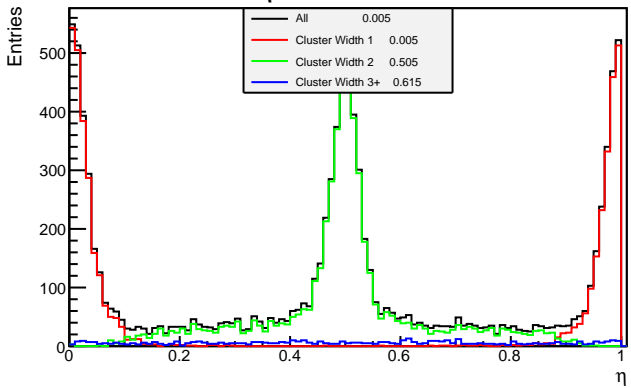
\eta -Distribution
