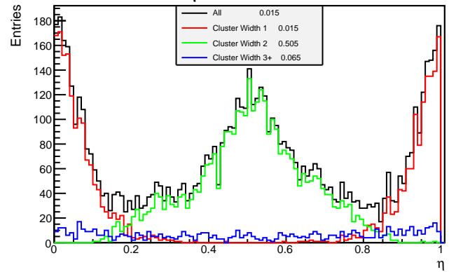
\eta -Distribution
