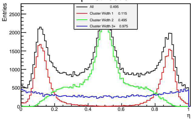
\eta -Distribution
